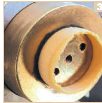
3 La filière en bronze ne modifie pas la structure des pâtes.
